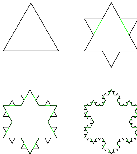
FIGURE 1 – Les quatre premiers polygones du flocon de Koch
